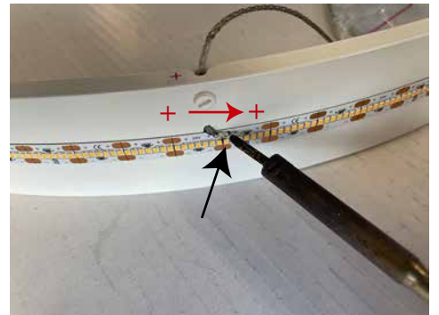
6 Lötkolben - Soldering iron - Fer à souder - Saldatore - Soldador + - - - +
