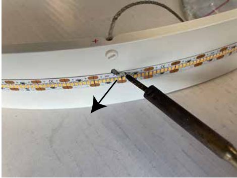
1 Lötkolben - Soldering iron - Fer à souder - Saldatore - Soldador
